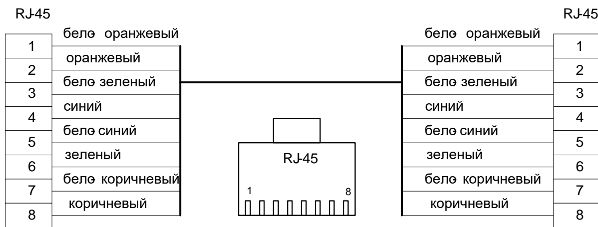
Рисунок 7.4 - Разделка кабеля.
